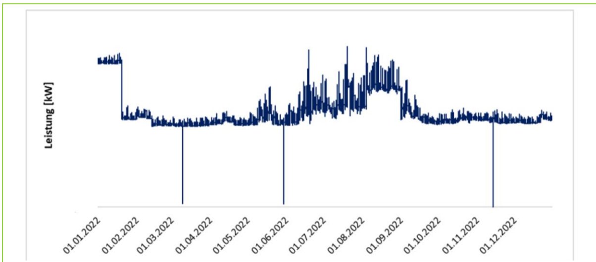
Abbildung 3: Lastkurve eines Aggregations-Standortes
