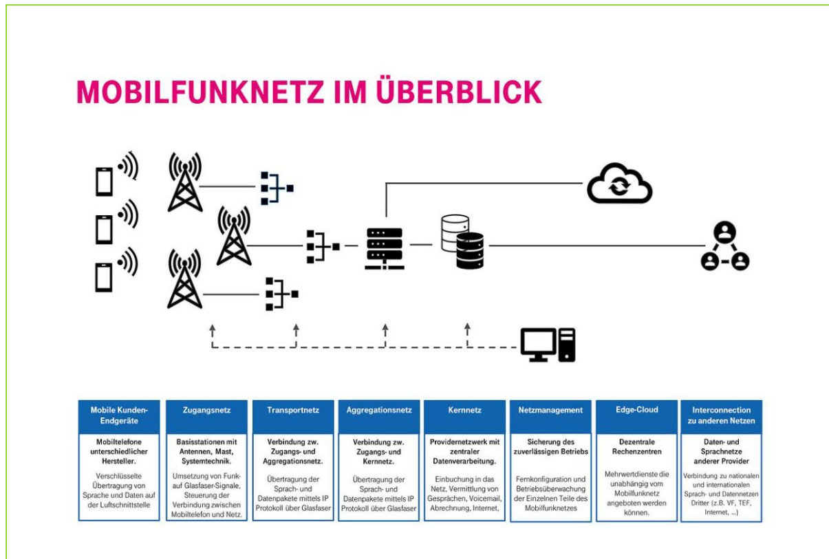
Abbildung 6: Mobilfunknetz im Überblick
