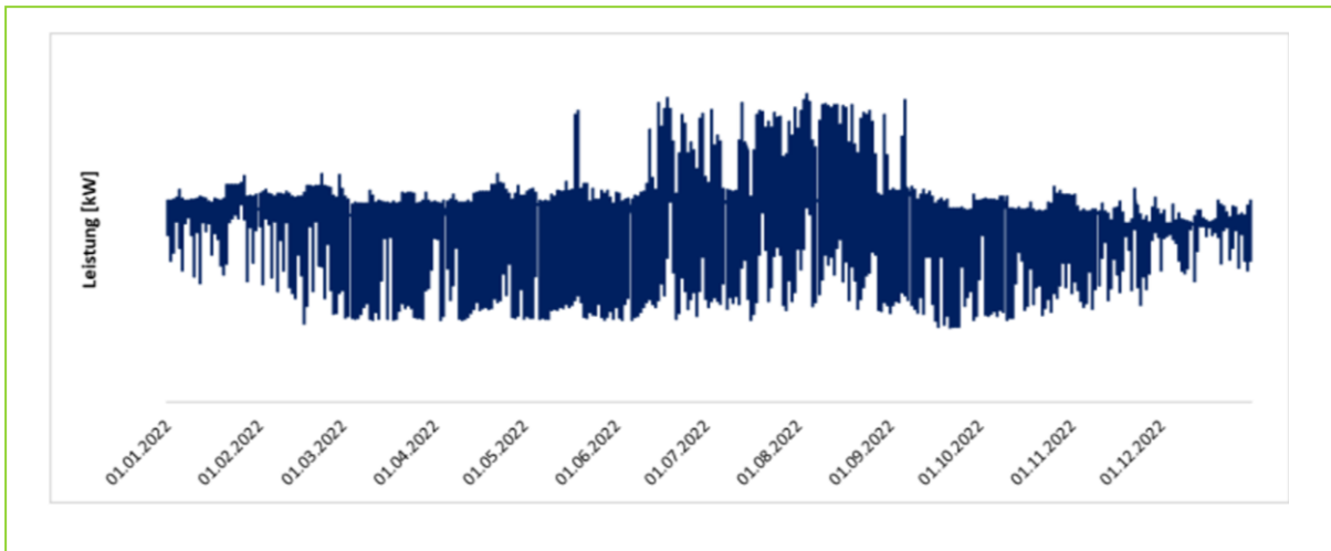
Abbildung 2: Lastkurve eines Access-Standortes
