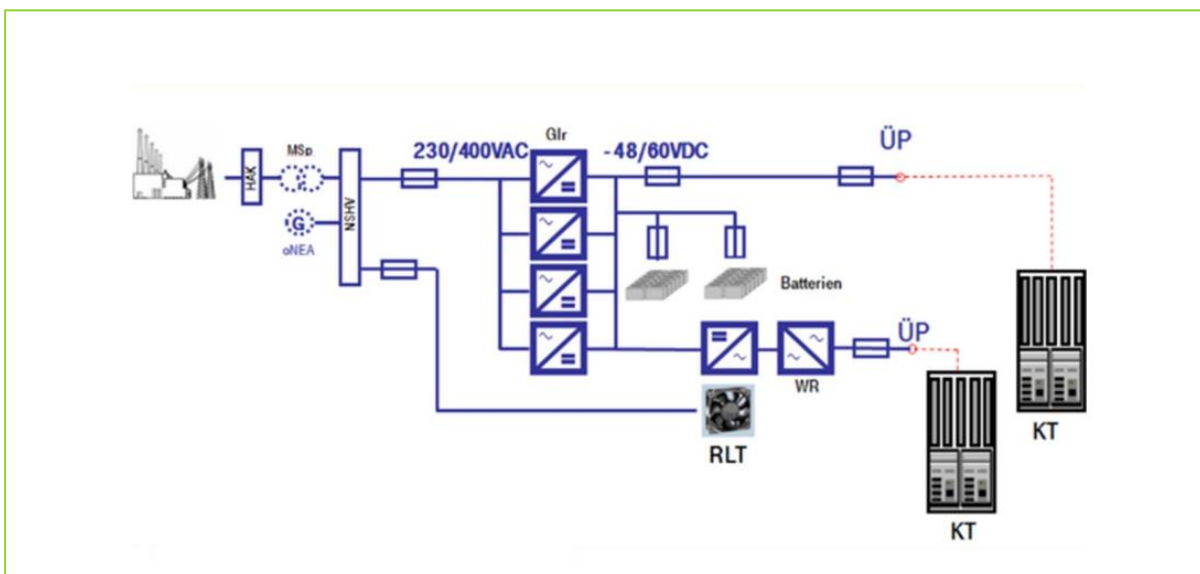
Abbildung 1: Typischer Aufbau der elektrischen Energieversorgung einer Betriebsstelle
