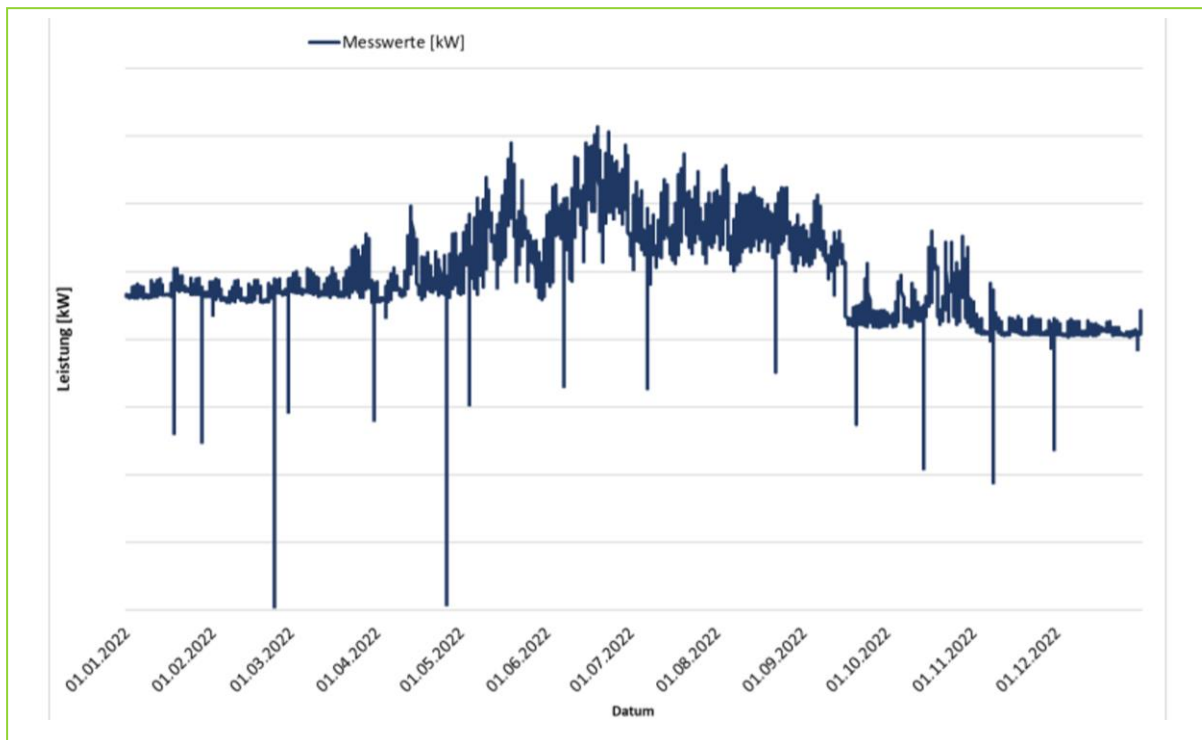
Abbildung 4: Lastkurve eines Core-Standortes
